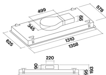
Dimensioni cappa e motore
